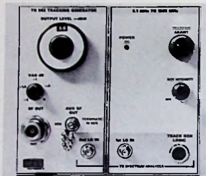
Eine Erweiterung der Serie 500 von Tektronix: der Mitlauf-Generator
