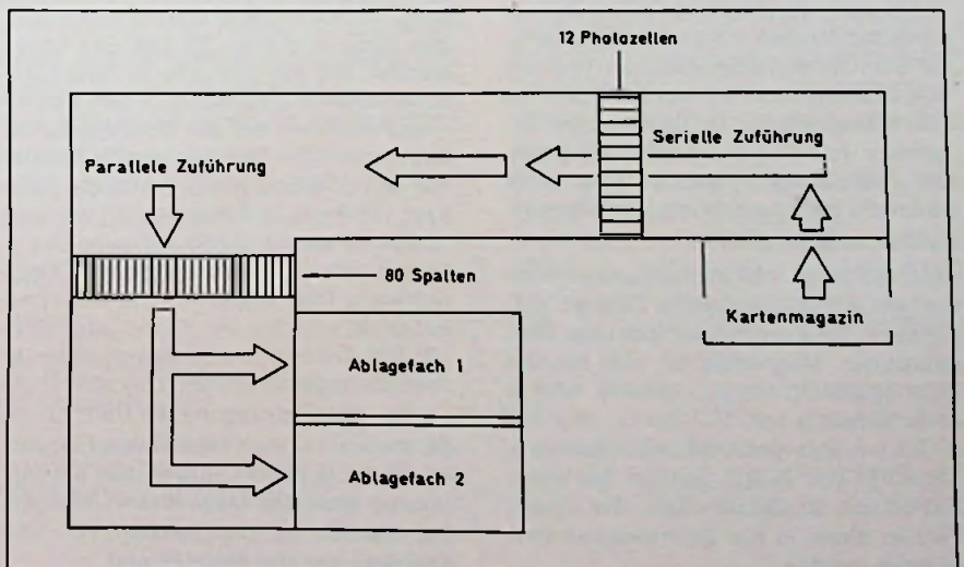
Diesen Weg legt die Lochkarte in einem Kartenleser zurück
