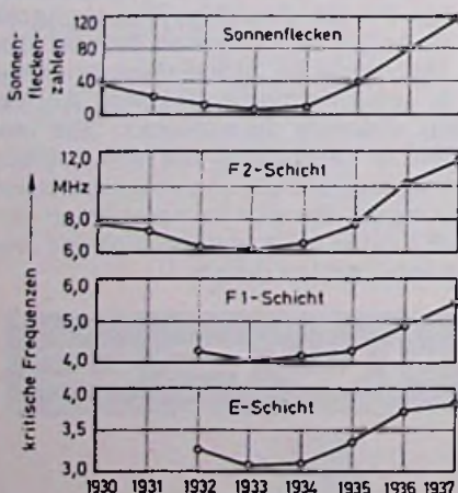
Vergleich der Jahresmittel der Sonnenfleckenzahl mit denen der Mittagswerte der kritischen Frequenzen der Ionosphärenschichten, ermittelt mit Hilfe der elektrischen Echolotung (die Schwankungen innerhalb eines Jahres sind der Einfachheit halber weggelassen worden)
